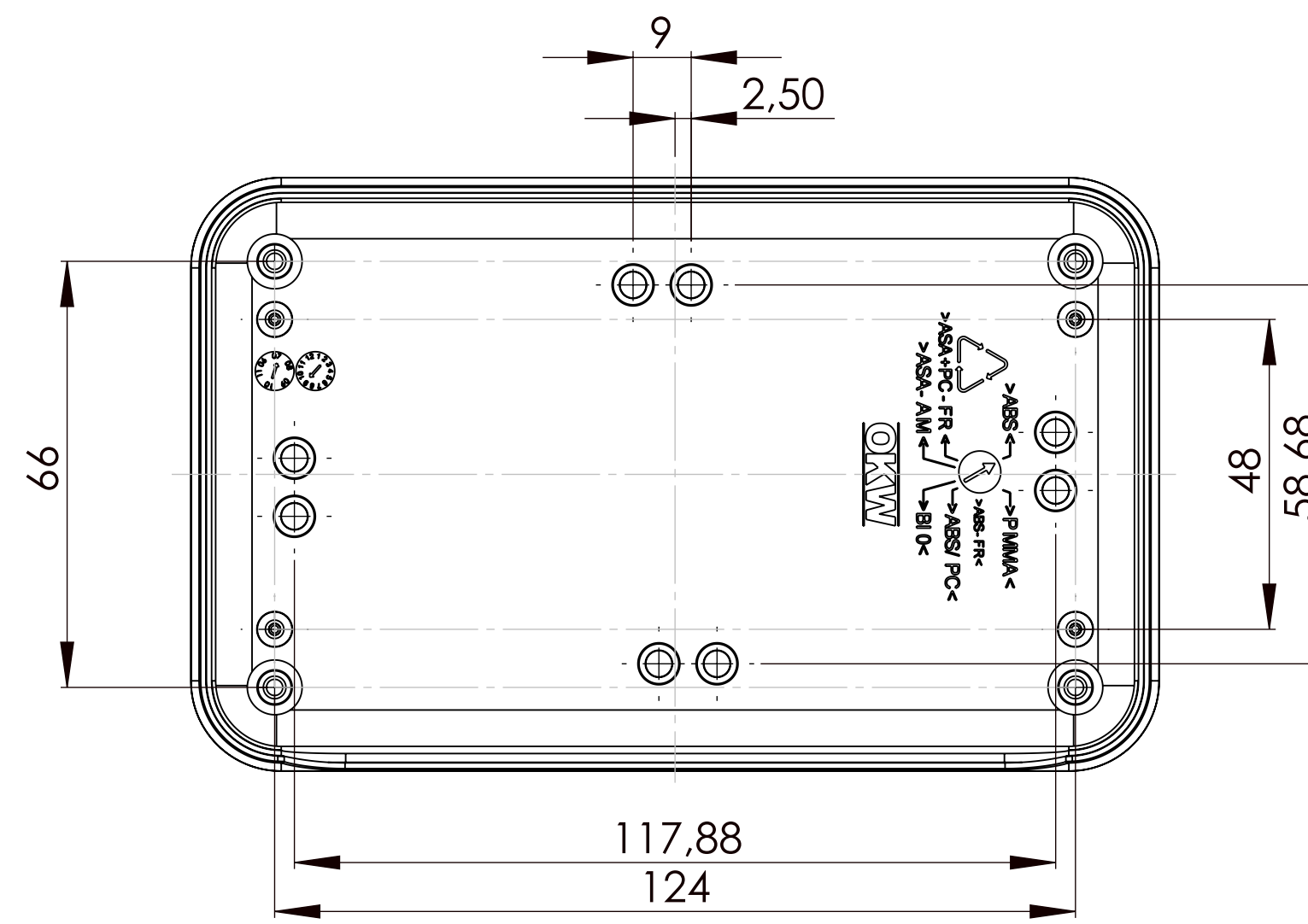
Unterteil Bottom-Part
