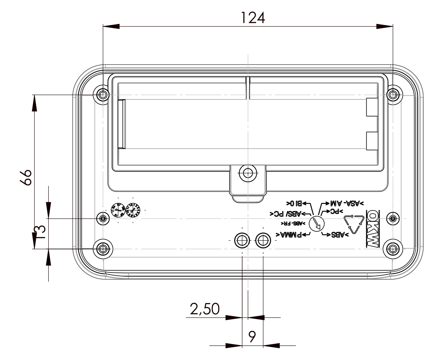
Unterteil mit Batteriefach 4x1,5V Bottom-Part with battery-compartment 4x1,5V
